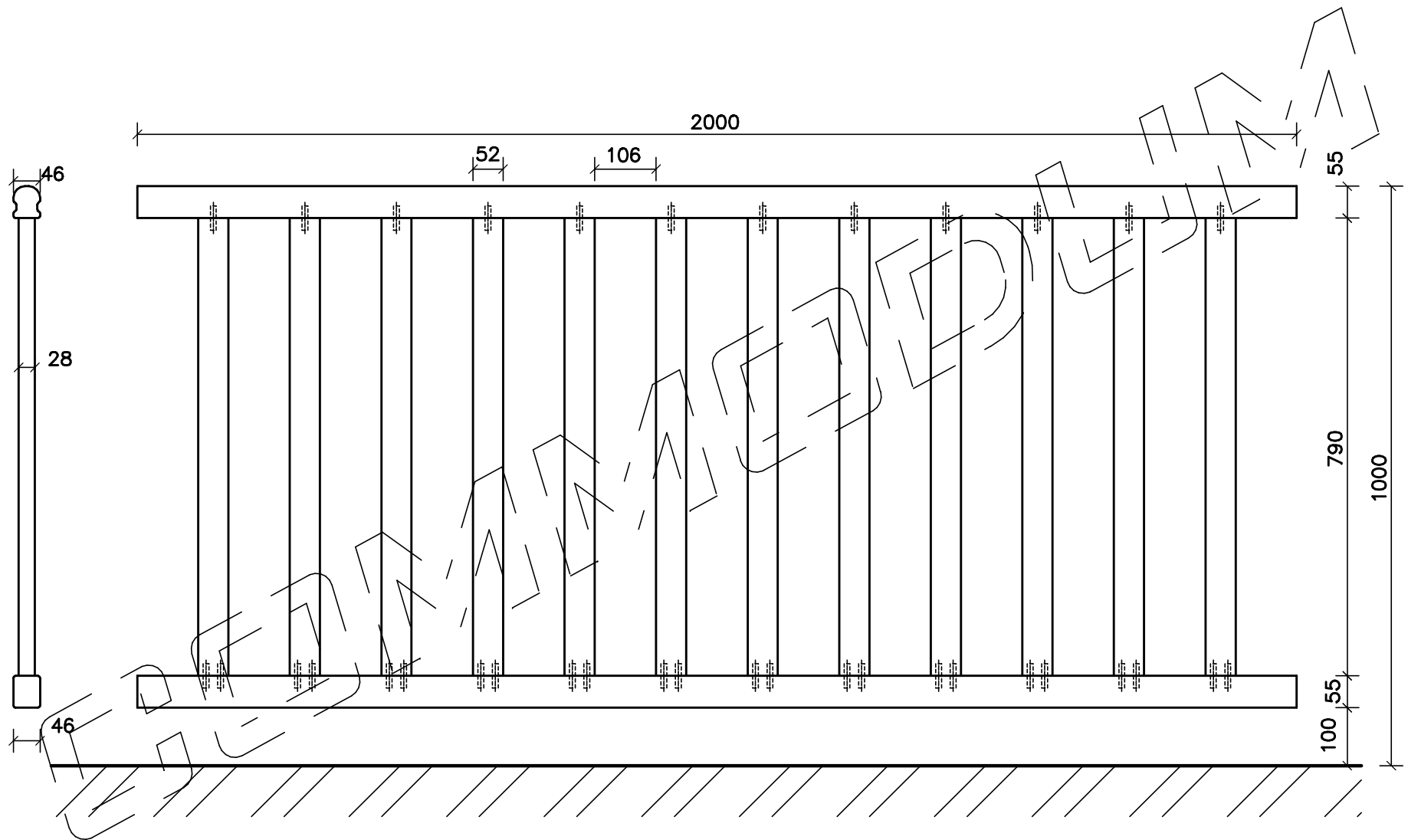
GALERIE 2000mm STANDARDNÍ SVISLÁ VÝPLŇ
