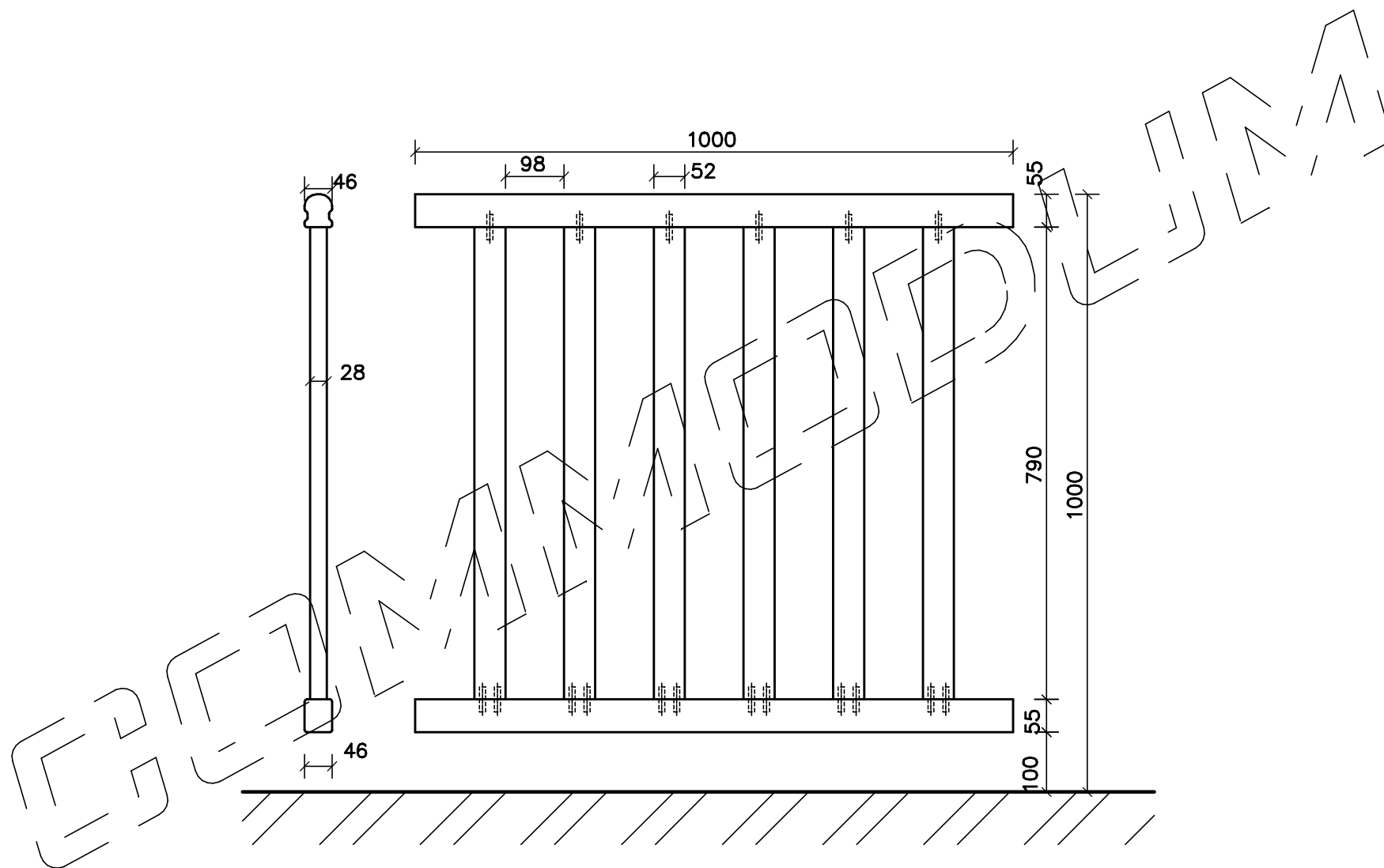
GALERIE 1000mm STANDARDNÍ SVISLÁ VÝPLŇ
