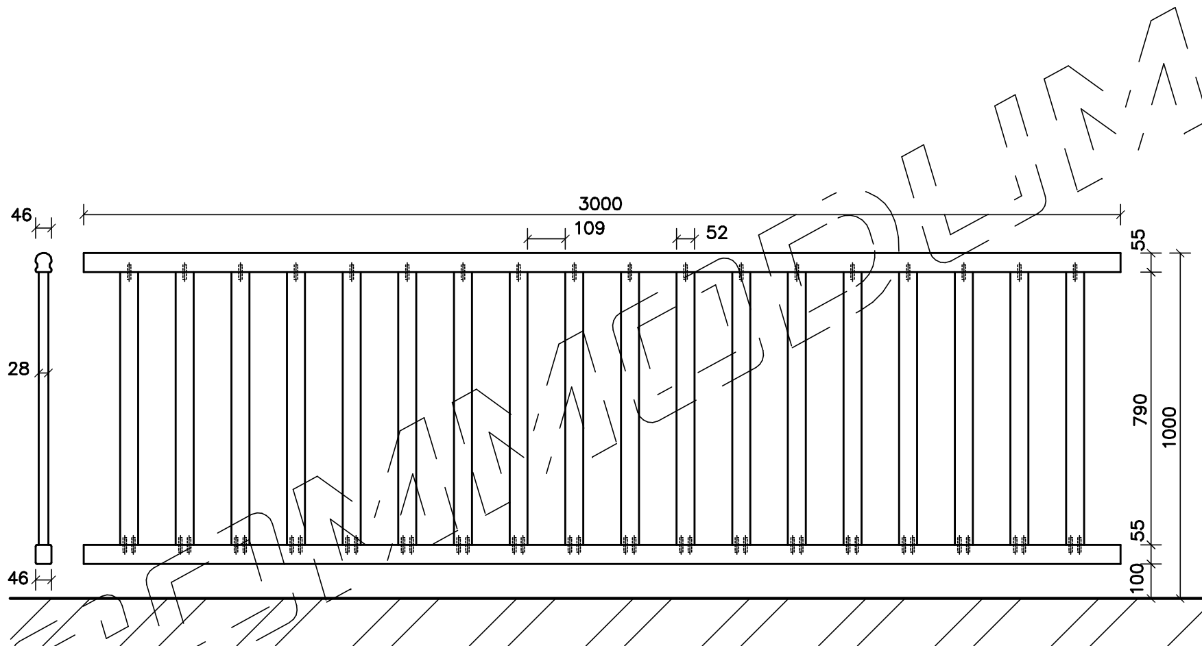
GALERIE 3000mm STANDARDNÍ SVISLÁ VÝPLŇ
